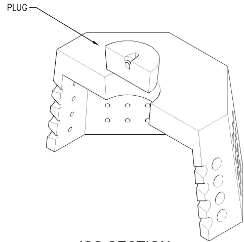
ISO SECTION SCALE: NTS
