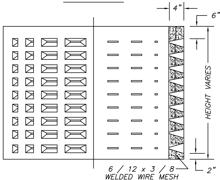
ELEVATION
